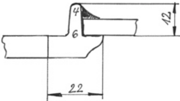
Fensterrahmen
