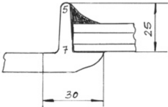
Fensterrahmen
