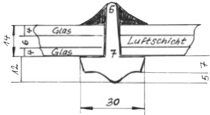
Innensteg
