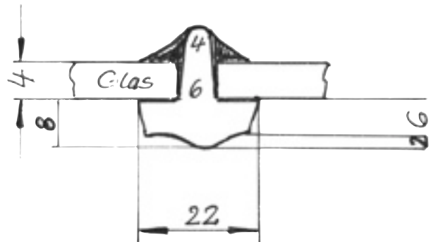
Innensteg
